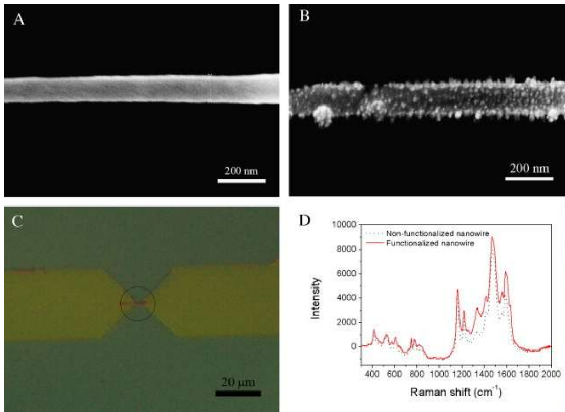
Fig. 1. (A) SEM obraz nemodifikovaného polyanilínového (PANI) nanovlákná (B) SEM obraz modifikovaného PANI nanovláka IgG protilátkou. (C) Modifikované PANI nanovláknko protilátkou IgG značený fluorescenční sondou Texas Red (v kroužku). (D) Srovnání Ramanova spektra před a po modifikaci PANI nanovlákná
